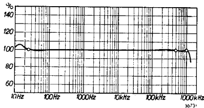
Fig. 2 Frequentiekarakteristiek
