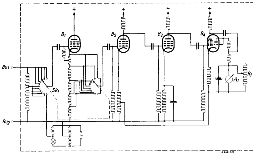
Fig. 1 Vereenvoudigd prinsieschema
