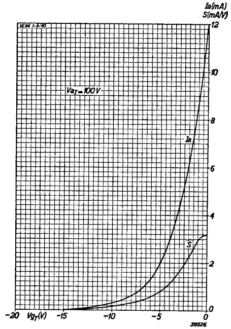
Fig. 15 Anodestroom en steilheit van het triodegedeelte als functie van de neg. roosterspanning bij V_{aT} = 100\ \text{V} .
