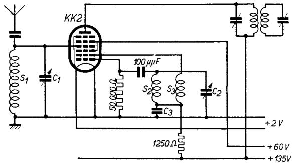
Schaltungsbeispiel ohne Patentbligo unsererseits. Prinzipschaltung für die Verwendung der KK2 auf Kurzwellen.
