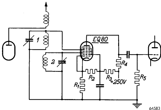
Fig. 4 Schéma de principe du tube EQ 80 utilisé comme détecteur F.M.
