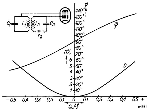
Fig. 5 Angle de phase \varphi et distortion totale D en fonction du rapport Q_2 \Delta f/f .
